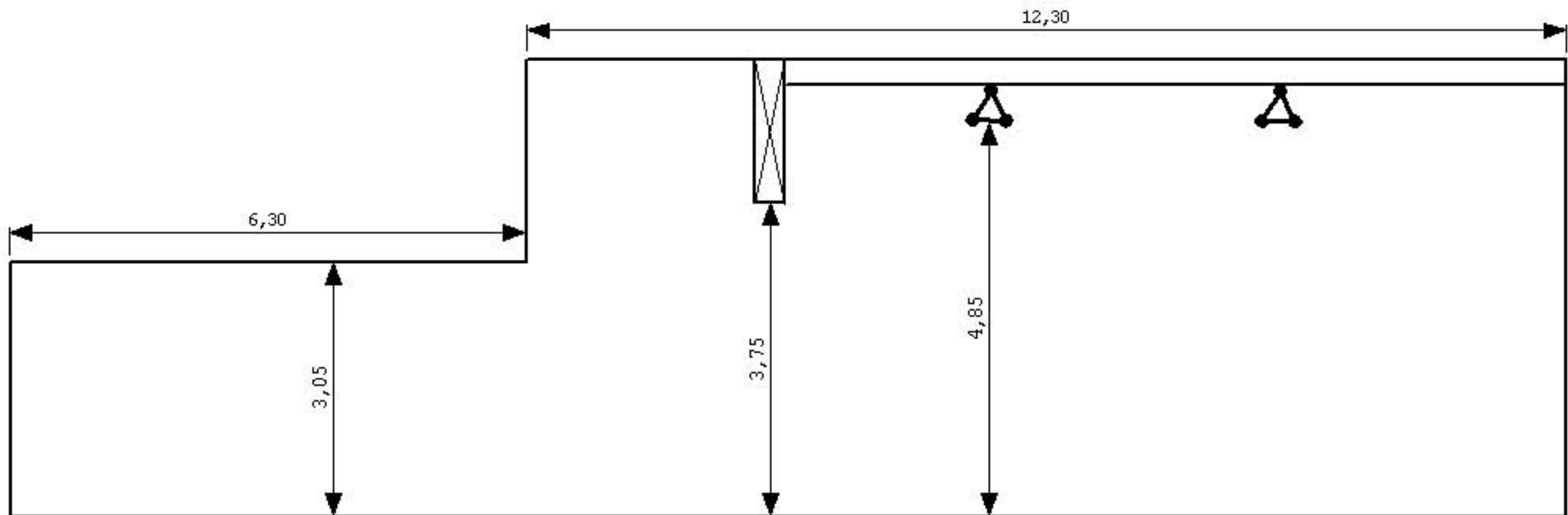
Theaterhaus Frankfurt Saal/Schnitt (alle Angaben in Meter)
